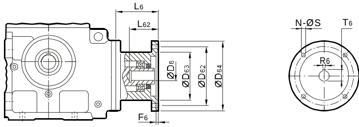
联结法兰尺寸 Adapter dimensions
